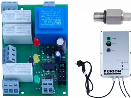
Bild: OPD 2 Platine, Sensor und Integration in Schaltkasten 2
